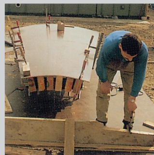
WEHA®-Trichterelement mit Betoplan belegt
